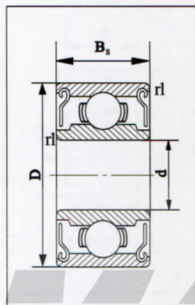
ZZ & 2RS
