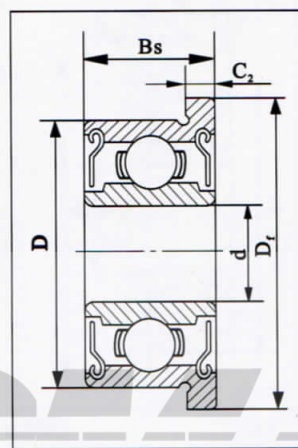
ZZ & 2RS
