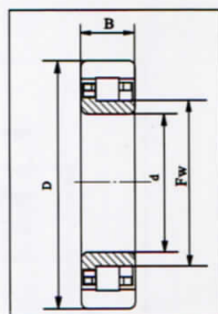
NJ 000
