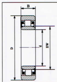
NU 000
