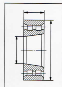
NN...K
