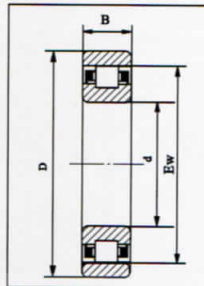
NF 000
