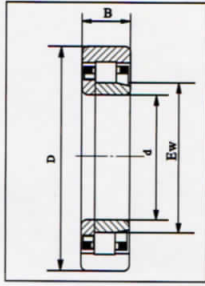
NUP 000
